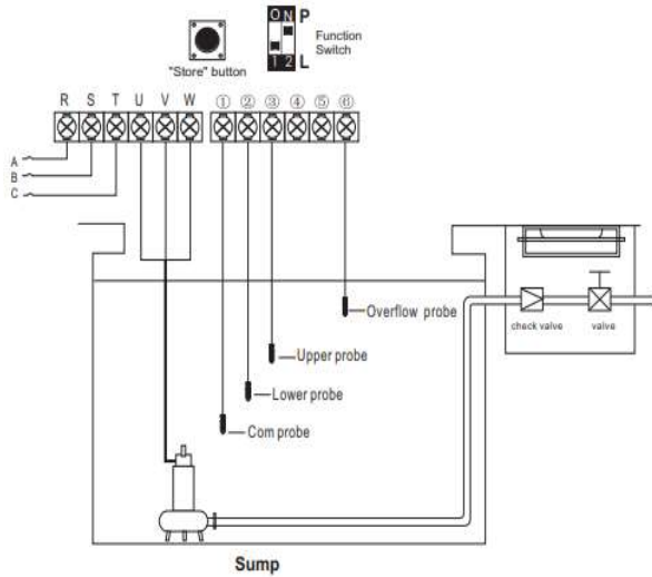
รูป 3.3.1.1. การต่อสายโพรบควบคุมบ้มนุ่ม
