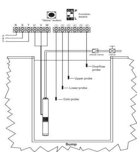
รูป 3.3.1.3. การต่อสายโพรบควบคุมบ้มนบาดาล
