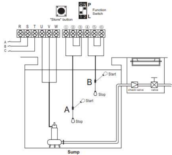
รูป 3.3.1.2. การต่อสวิตช์ลูกลอยควบคุมบ้มนุ่ม
