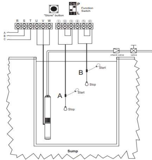
รูป 3.3.1.4. การต่อสวิตช์ลูกลอยควบคุมบ้มนบาดาล
