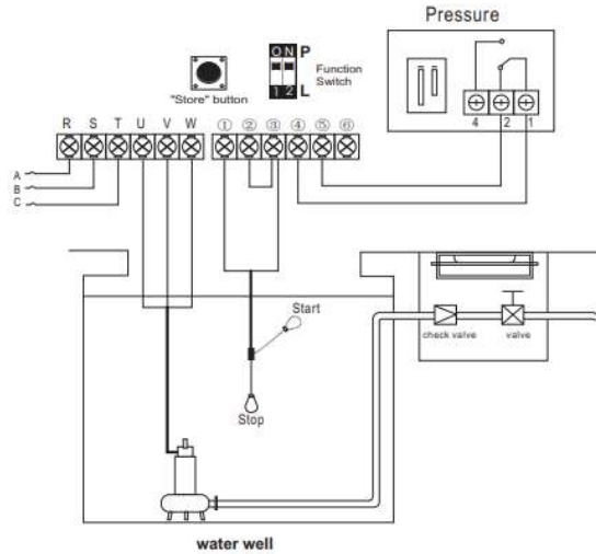
รูป 3.3.1.2. ต่อลูกลอย & สวิทช์แรงดันควบคุมบีมจุ่ม
