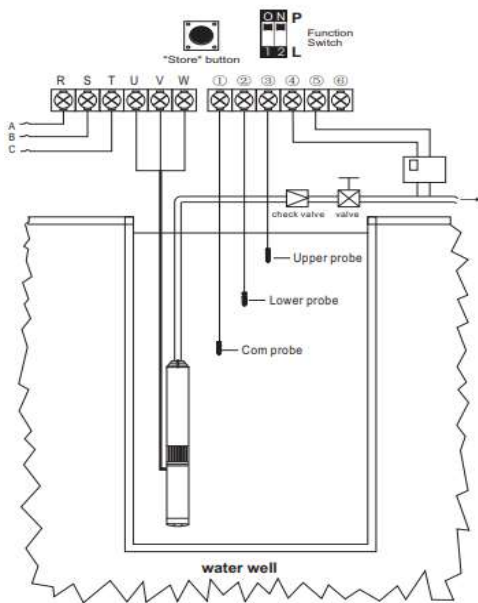
รูป 3.3.1.3. ต่อสายโพรบ & สวิทช์แรงดันควบคุมบีมบาดาล
