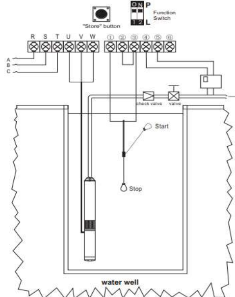
รูป 3.3.1.4. ต่อลูกลอย & สวิทช์แรงดันควบคุมบีมบาดาล
