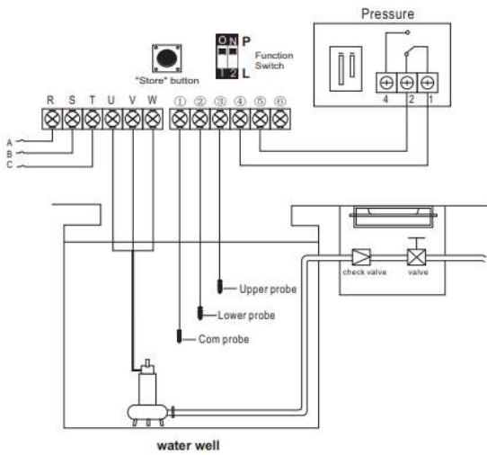
รูป 3.3.1.1. ต่อสายโพรบ & สวิทช์แรงดันควบคุมบีมจุ่ม
